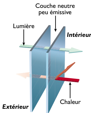
Double Vitrage à Isolation Renforcée
